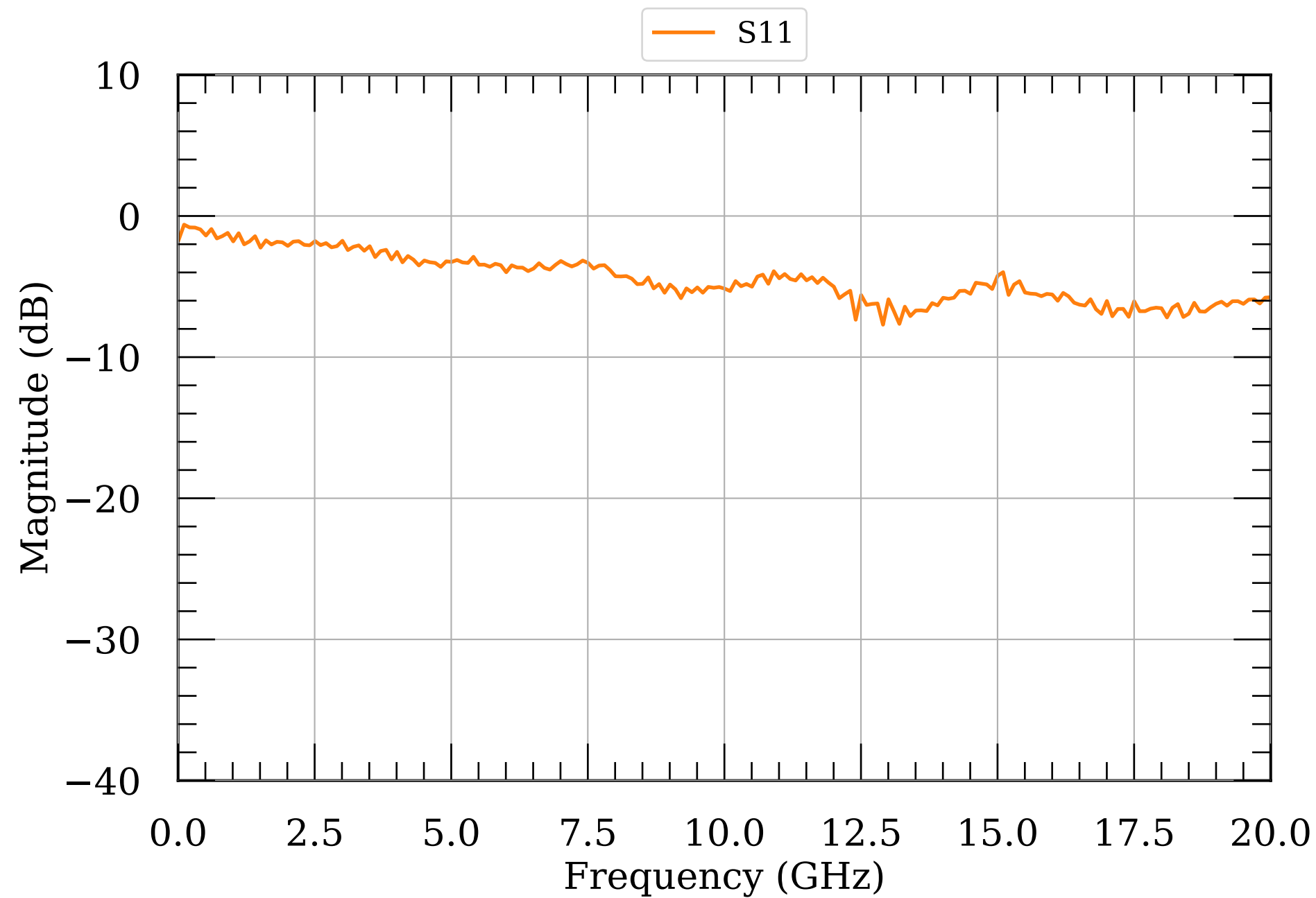
LNA S-params module065
